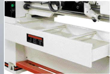
Ausziehbare Spänewanne
